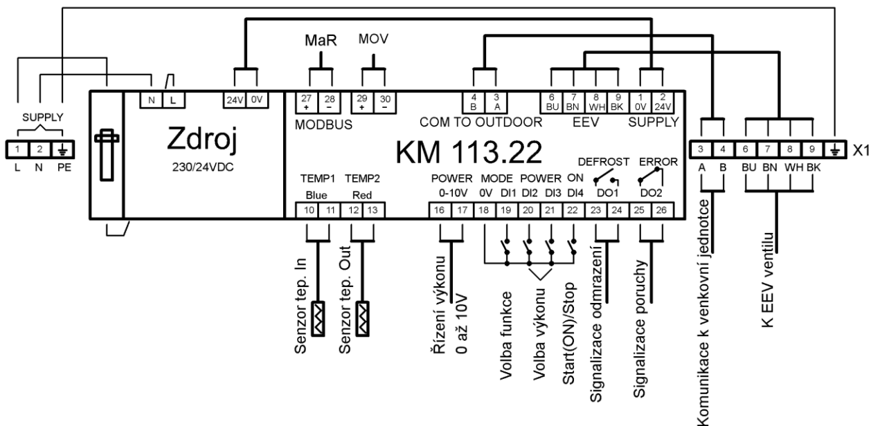
Obr. 2 CELKOVÉ SCHÉMA SVOREK
