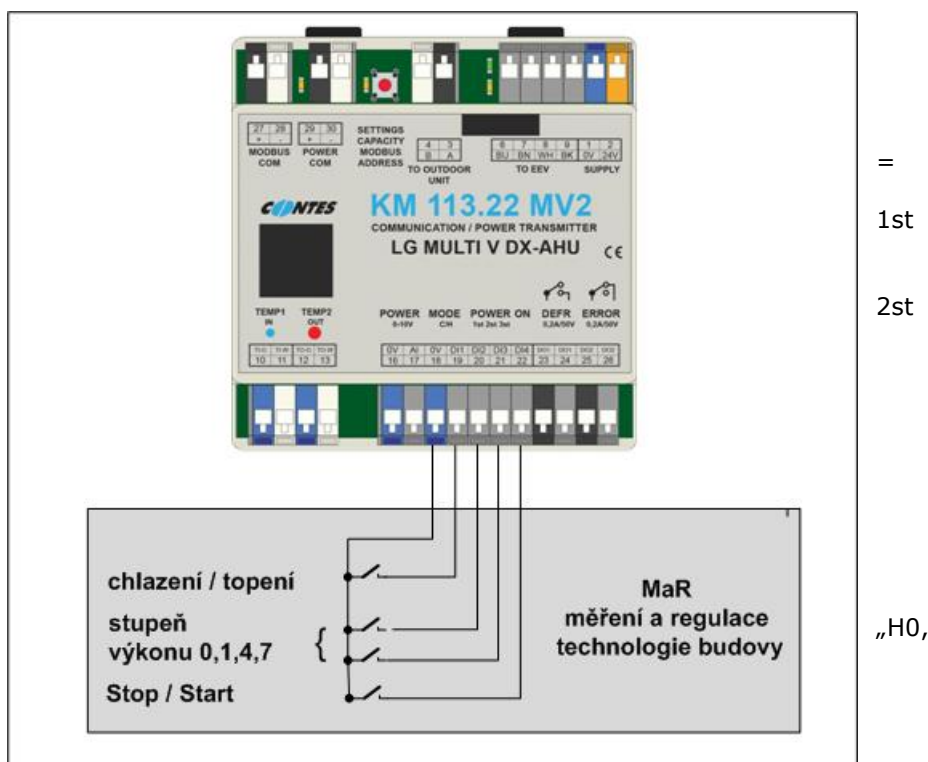
Obr.5 SCHEMA OVLÁDÁNÍ LOGICKÝMI SIGNÁLY - TYPU VOLNÝ KONTAKT
