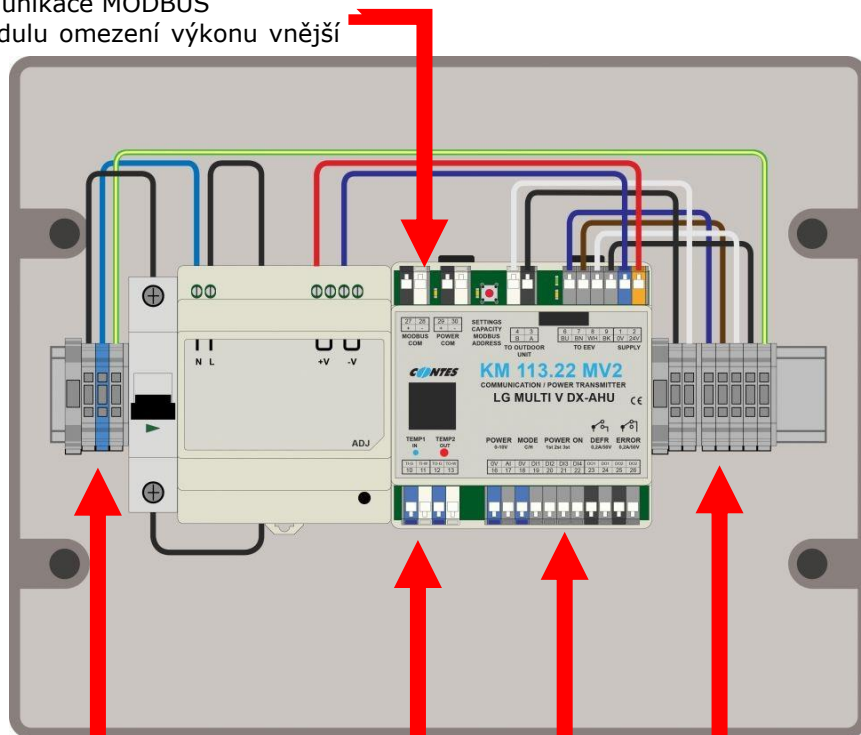
Obr. 3 ROZDĚLENÍ SVOREK MODULU KM113.22MV2
