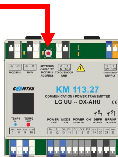
Obr.9 SCHÉMA AKTIVACE NASTAVOVACÍHO REŽIMU
